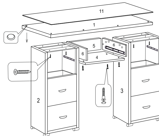
Рис.4 Сборка стола
